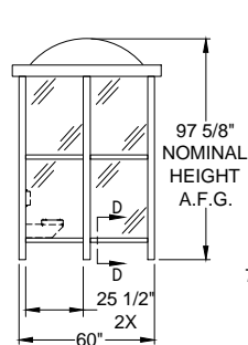
ELEVATION B
